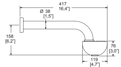
Dimensiones: vista frontal
