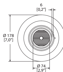
Dimensiones: vista cenital
