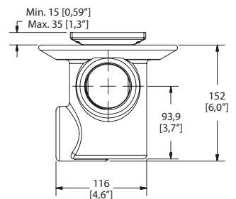
Dimensiones: vista lateral
