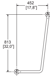
Dimensiones: vista frontal
