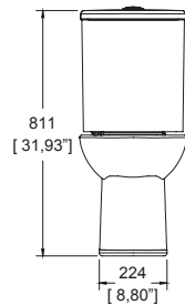
Dimensiones: vista frontal
