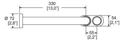
Dimensiones: vista cenital
