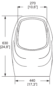
Dimensiones: vista frontal
