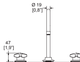
Dimensiones: vista frontal
