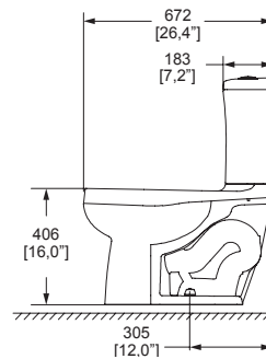
Dimensiones: vista lateral
