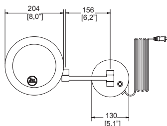
Dimensiones: vista frontal
