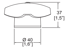
Dimensiones: vista lateral
