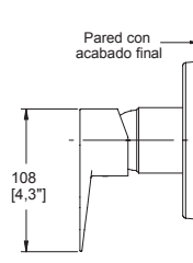
Dimensiones: vista lateral
