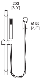
Dimensiones: vista frontal
