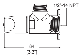
Dimensiones: vista lateral
