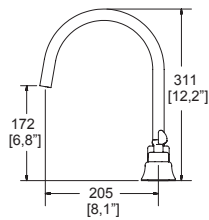
Dimensiones: vista lateral
