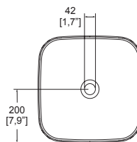
Dimensiones: vista cenital
