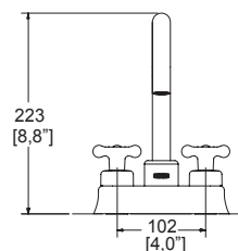
Dimensiones: vista frontal
