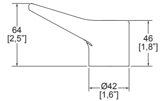
Dimensiones: vista lateral
