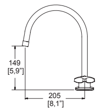
Dimensiones: vista lateral
