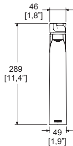
Dimensiones: vista frontal
