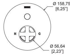
Dimensiones: vista frontal
