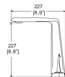
Dimensiones: vista lateral
