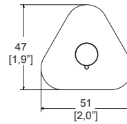
Dimensiones: vista frontal
