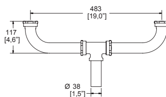
Dimensiones: vista frontal
